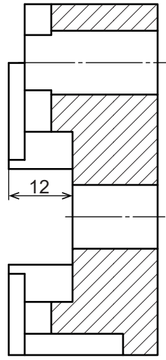
A-A'
