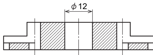
A-A' (断面部分にハッチング処理)
