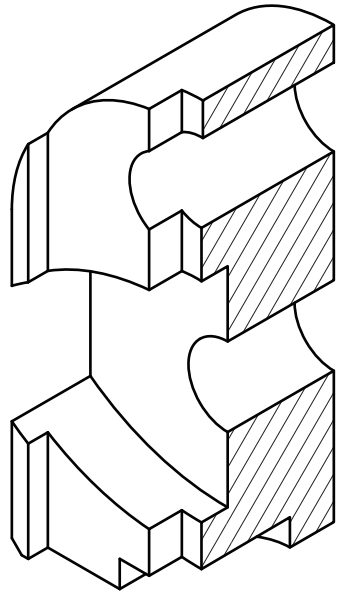
A-A' 断面图
